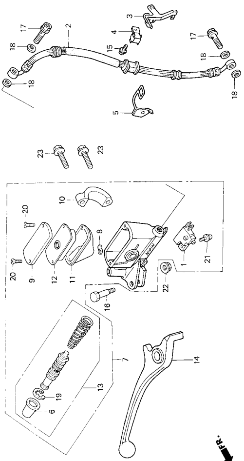
F - 4 แม่ปั๊มเบรคหน้า Front Brake Master Cylinder (NF100D, MD)
