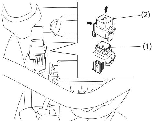
(1) PS fuse
