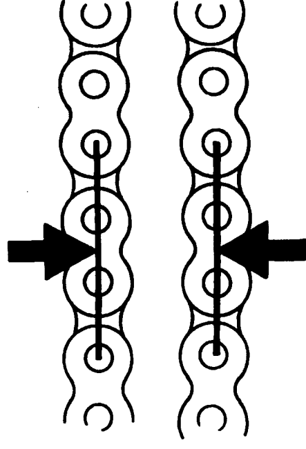
ドライブチェーンの緩み(たるみ)
