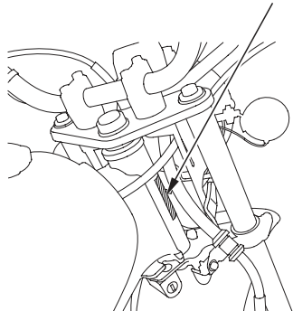
フレーム号機打刻位置
