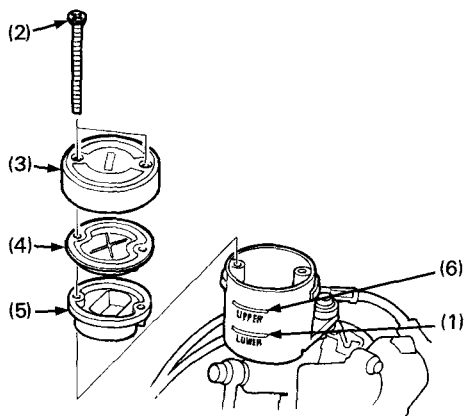
(2) Schrauben (5) Membran (3) Reservoirdeckel (6) Obere Markierung (4) Membranplatte (UPPER)
